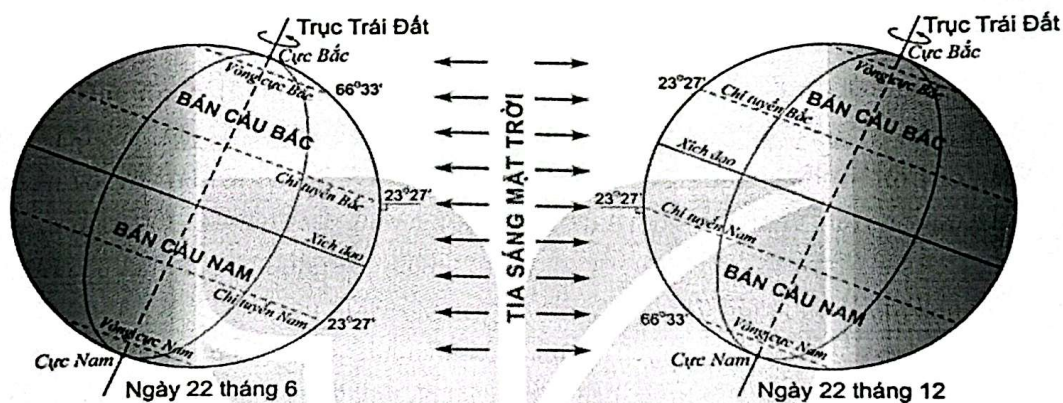
Hình 2. Góc chiếu của tia sáng mặt trời tới Trái Đất
