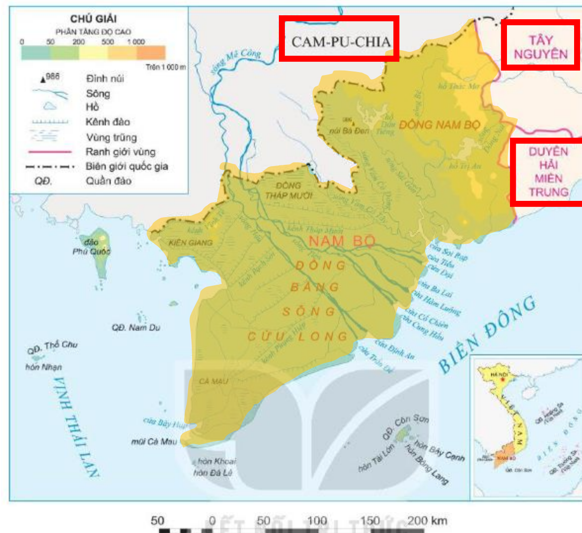
Hình 1. Lược đồ địa hình vùng Nam Bộ
