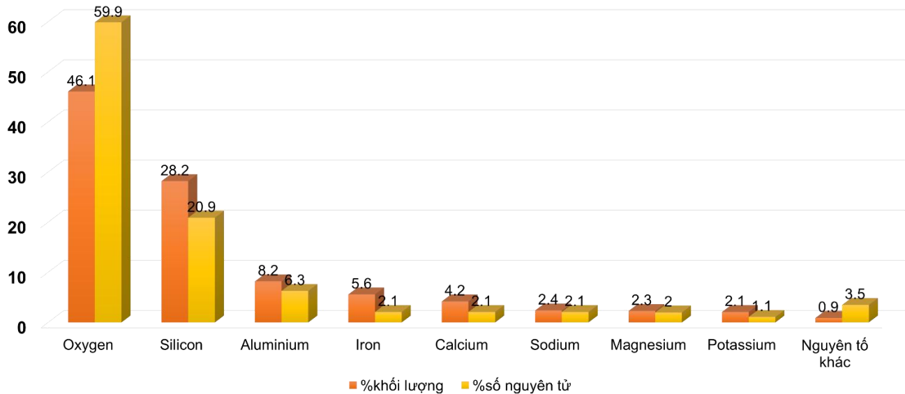
Biểu đồ mô tả tỉ lệ phần trăm của một số nguyên tố hóa học trong lớp vỏ Trái Đất
