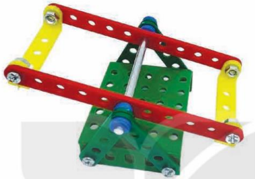
Hình 4 Mô hình bập bênh hoàn thiện
