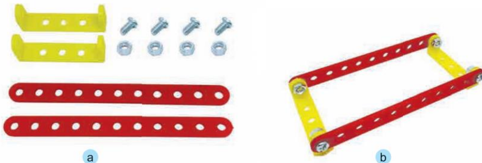
Hình 3 Các chi tiết và ghế ngồi tập thể dục
